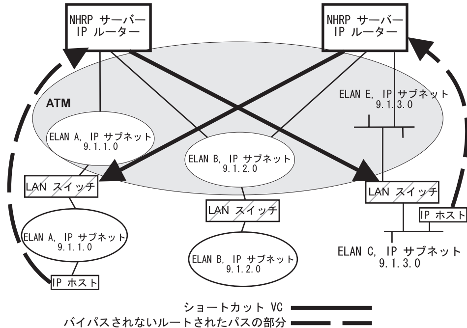
図 32. LAN スイッチをもつ ELAN 環境における NHRP
