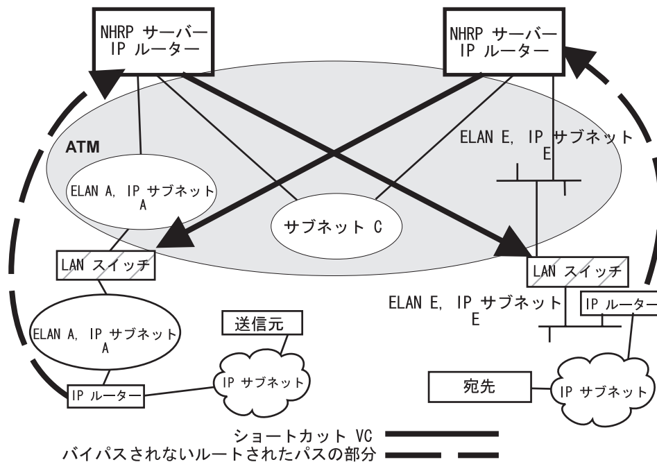
図 34. 出口ルーターへの NHRP
