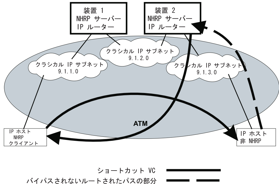
図 30. 非 NHRP 装置をもつクラシカル IP 環境における NHRP
