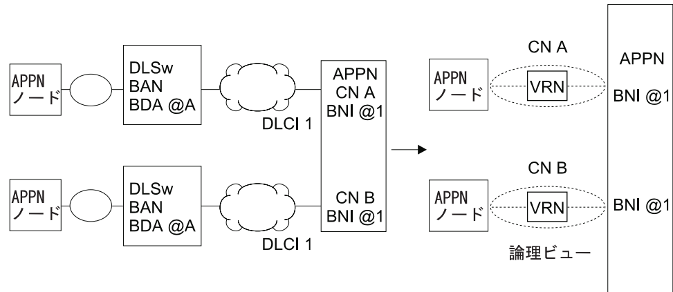
図9. BAN を使用する複数の接続ネットワーク
