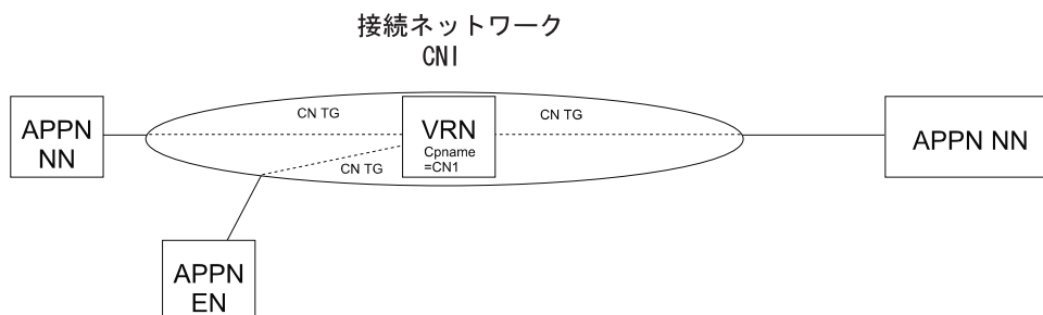
図6. APPN フレーム・リレー・ブリッジ・フレーム/BAN 接続ネットワーク
