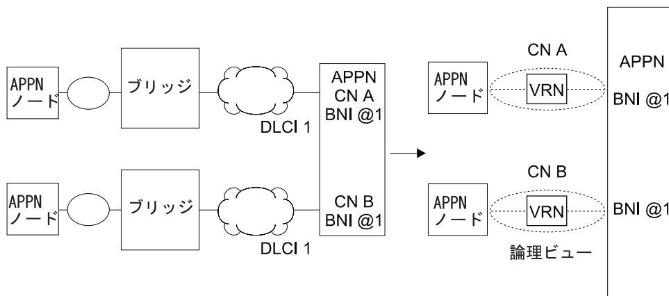
図 12. ブリッジングを使用する複数の接続ネットワーク
