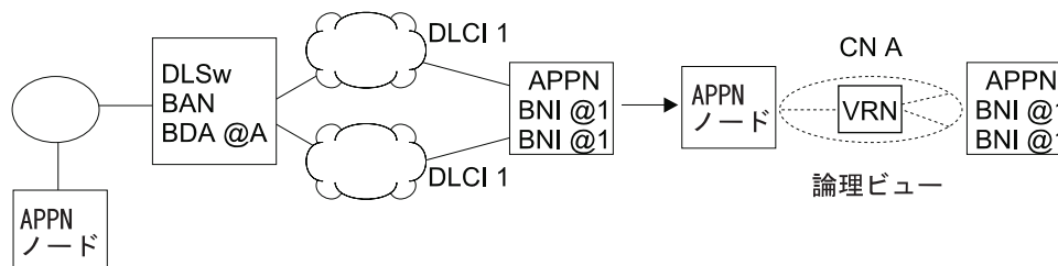
図8. BAN と複数のフレーム・リレー・ポートを使用する単一接続ネットワーク
