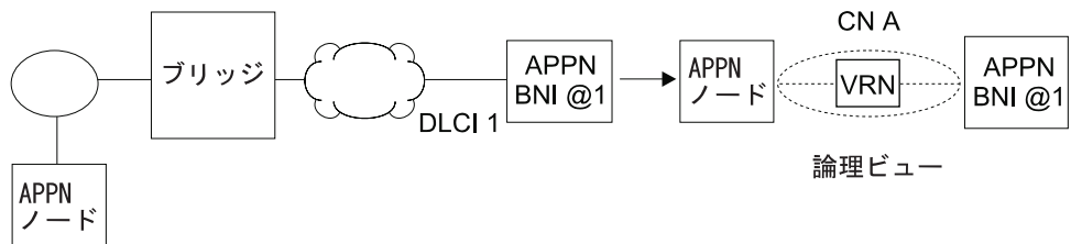
図10.ブリッジングと1つのフレーム・リレー・ポートを使用する単一接続ネットワーク
