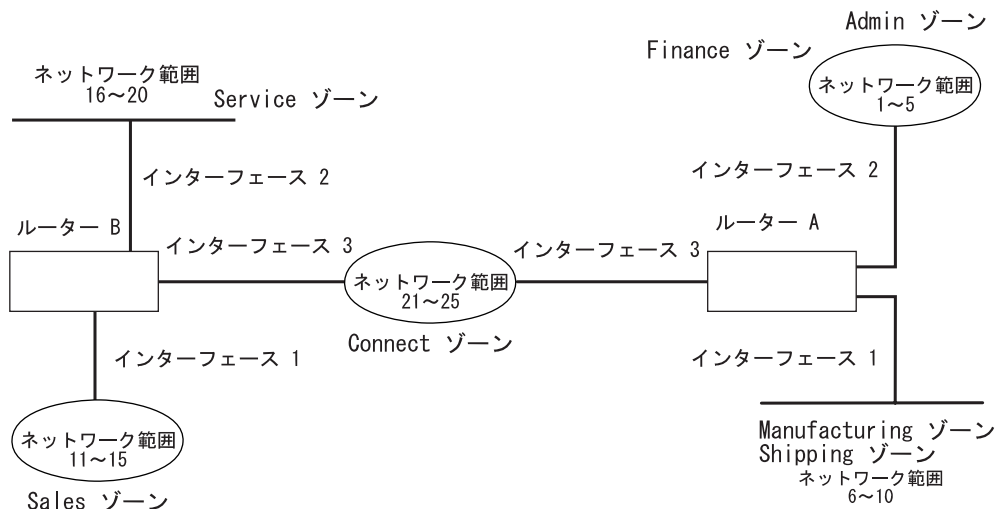
図 14. ネットワーク・フィルターの例.
