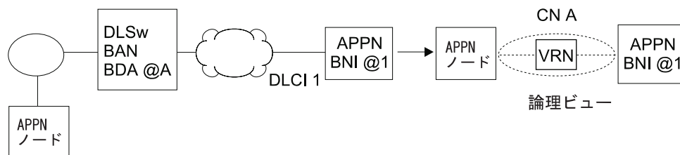
図7. BAN と 1 つのフレーム・リレー・ポートを使用する単一接続ネットワーク
