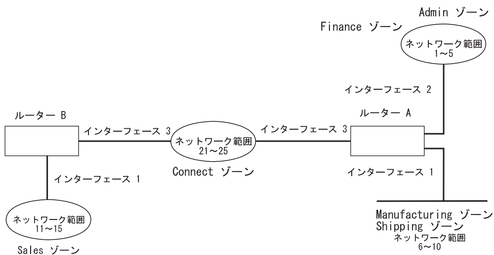
図 13. ゾーン・フィルターの例
