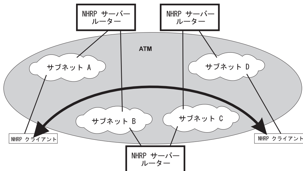
クライアント間トラフィックのショートカット VC
