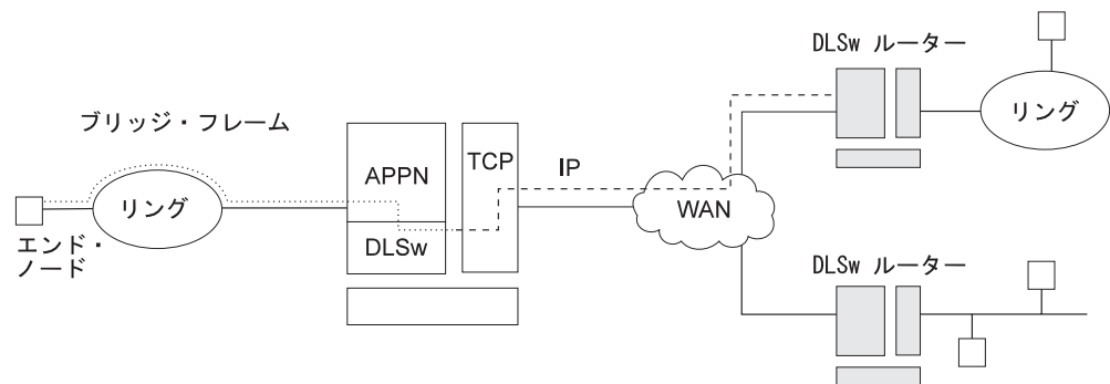
図4. DLSw ポートを使用する APPN 構成のデータの流れ
