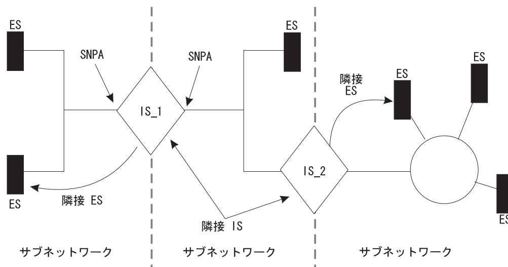
図 21. OSI ネットワーク
