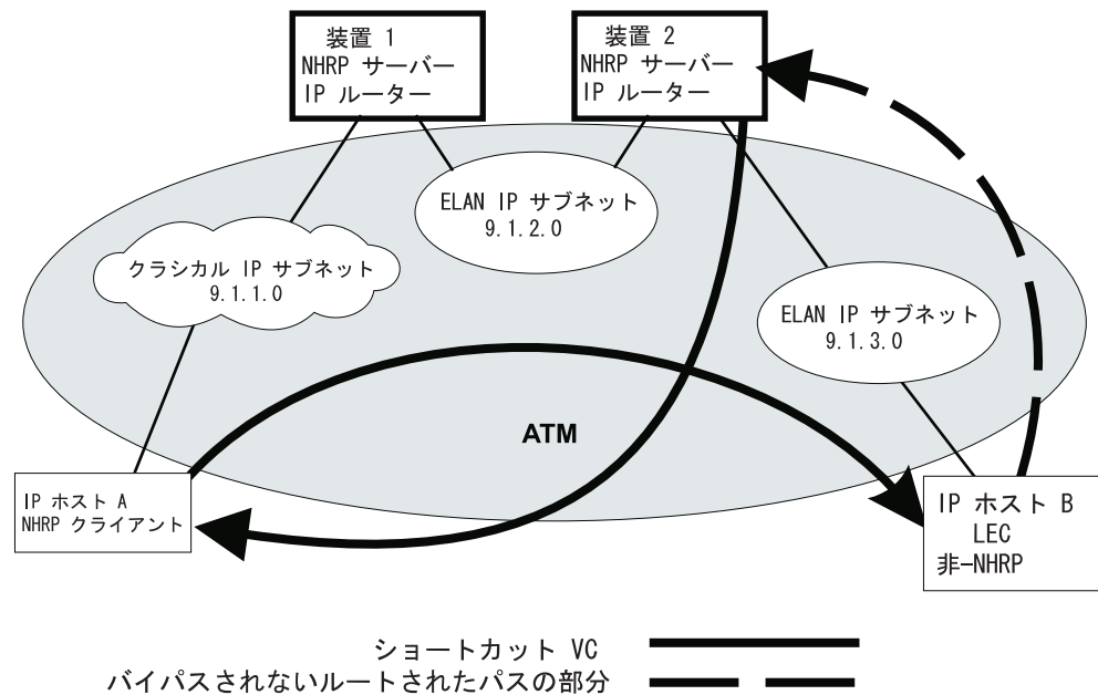
図 33. 混合されたクラシカル IP および ELAN 環境における NHRP
