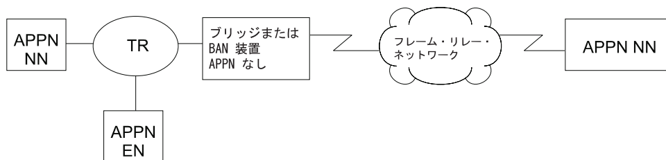
図5. フレーム・リレー・ブリッジ・フレーム/BAN 接続ネットワーク・サポートを使用した場合の論理ビュー
