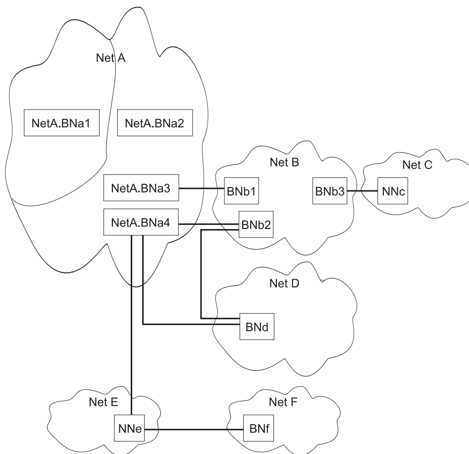
図2. 拡張ボーダー・ノードの接続
