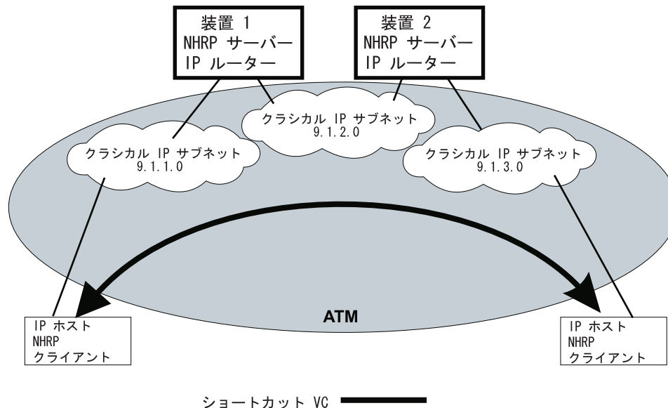
図 29. クラシカル IP 環境における NHRP
