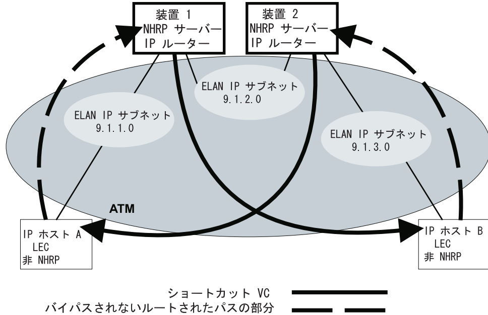
図 31. ELAN 環境における NHRP
